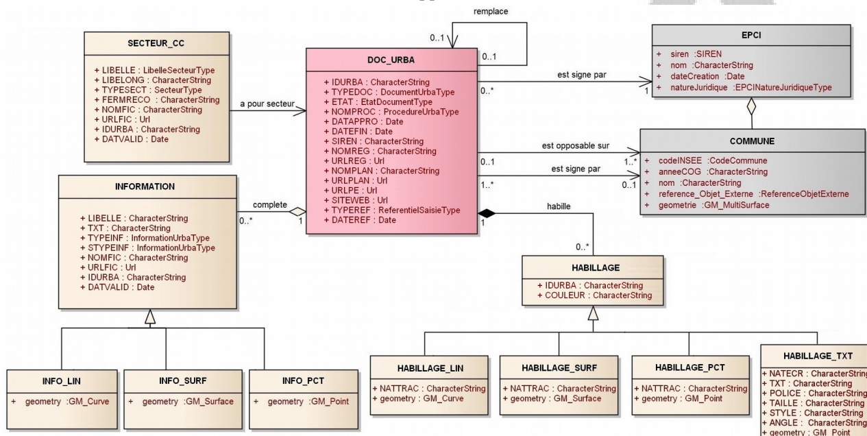
Les différentes classes et leurs relations représentées en UML
