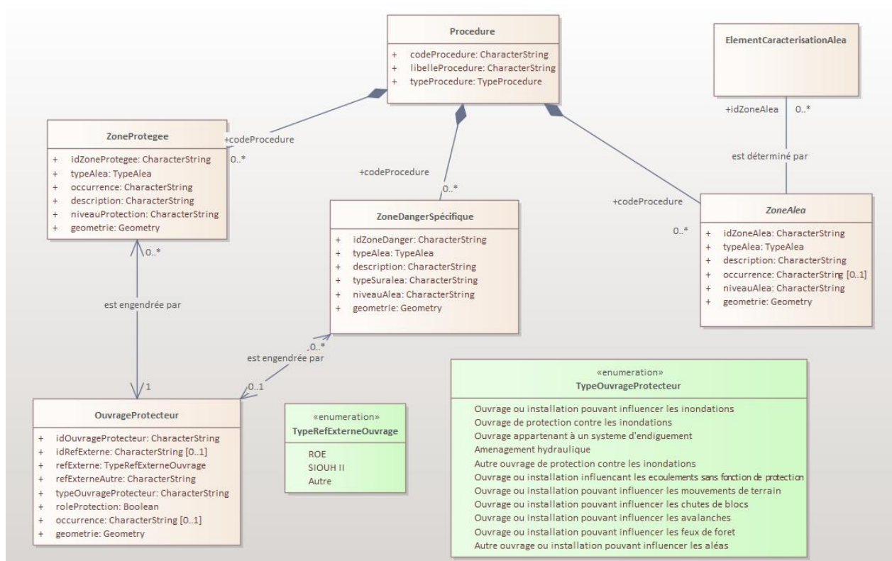
Figure 3 - Modèle UML des classes relatives aux aléas.
