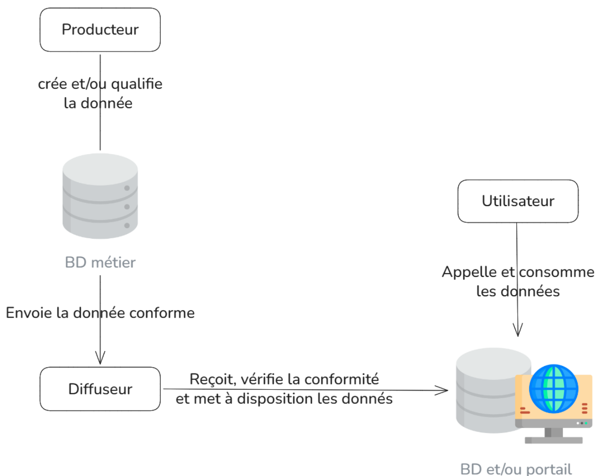
Figure 1 - Schéma de cas d'usage du standard
