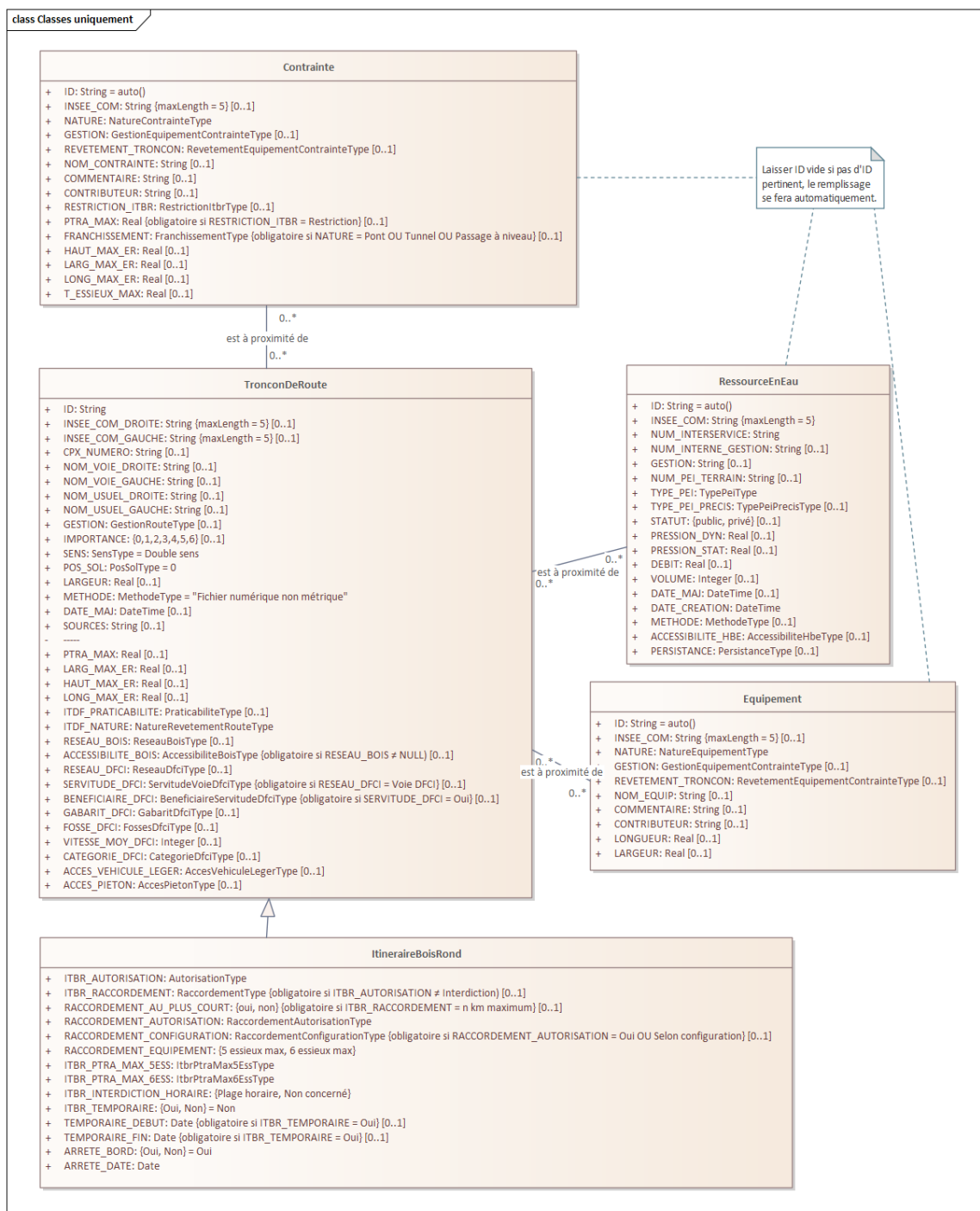
Figure 2 : Diagramme de classe (sans les énumérations)
